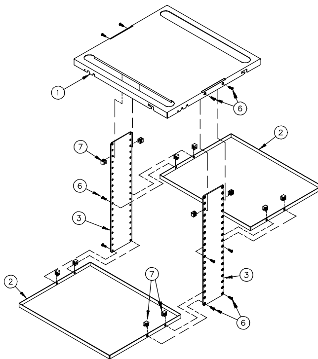
600mm Deep Shelf in 600mm Frame 600mm tiefes Regal im 600mm Rahmen étagère profonde de 600mm dans l'armature de 600mm estante profundo de 600m m en el marco de 600m m
