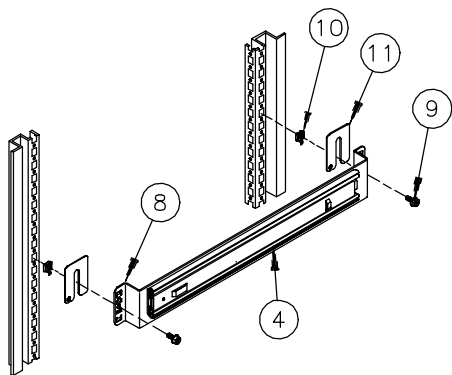
600mm Deep Shelf in 600mm Frame 600mm tiefes Regal im 600mm Rahmen étagère profonde de 600mm dans l'armature de 600mm estante profundo de 600m m en el marco de 600m m
