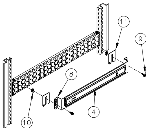
800mm Deep Shelf in 800mm Frame 800mm tiefes Regal im 800mm Rahmen étagère profonde de 800mm dans l'armature de 800mm estante profundo de 800m m en el marco de 800m m
