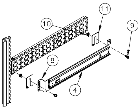
600mm Deep Shelf in 800mm Frame 600mm tiefes Regal im 800mm Rahmen étagère profonde de 600mm dans l'armature de 800mm estante profundo de 600m m en el marco de 800m m
